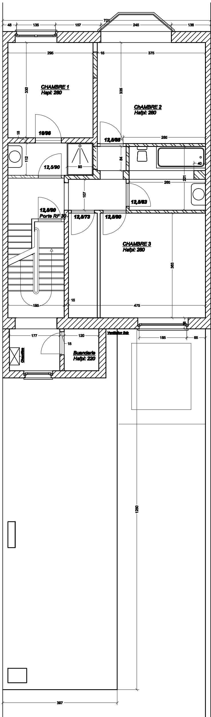
Vue en plan 2EME ETAGE Situation projetée
